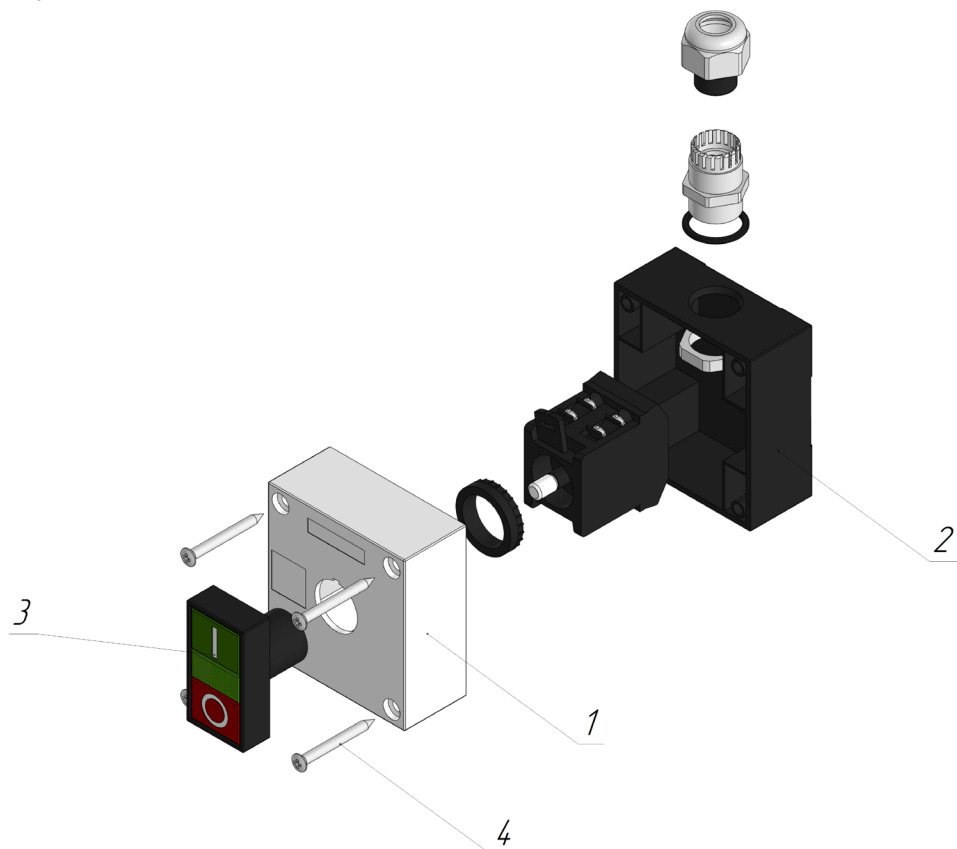
Рисунок 3.2.1 – 3D-модель ПУ-1-XYZ
