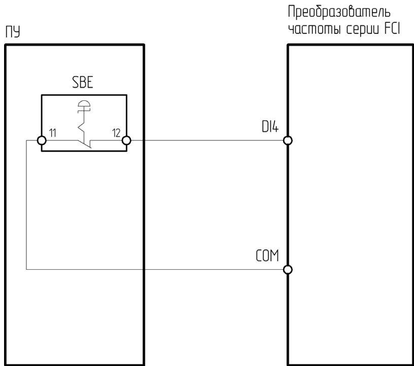
Рисунок 4.5.9 – Схема подключения ПУ-1-070 к преобразователю частоты серии FCI
