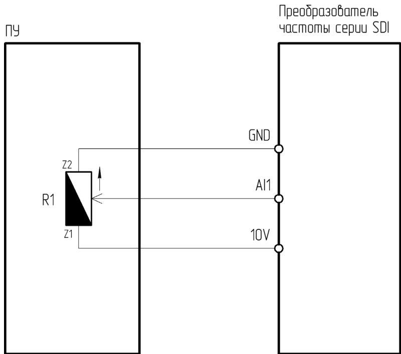
Рисунок 4.1.2 – Схема подключения ПУ-1-001 к преобразователю частоты серии SDI Таблица 4.1.2 – Настройка ПЧ серии SDI при подключении ПУ-1-001
