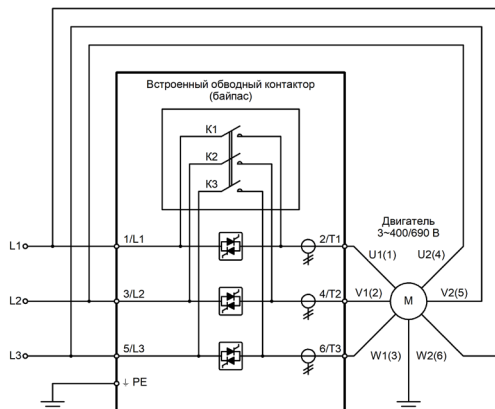
Схема подключения двигателя «внутри треугольника»
