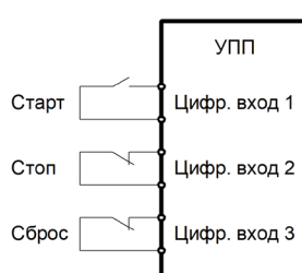
Четырехпроводное подключение
