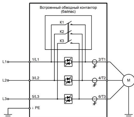
Схема подключения двигателя «в линию»
