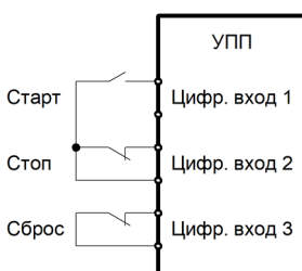
Трехпроводное подключение
