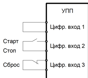
Двухпроводное подключение
