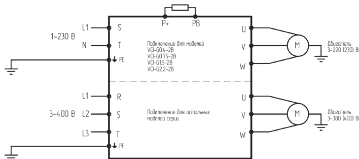
Рис 3.2 Схема силовых подключений
