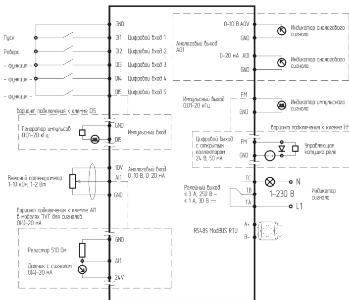
Рис. 3.4 – Схема подключения управляющих клемм
