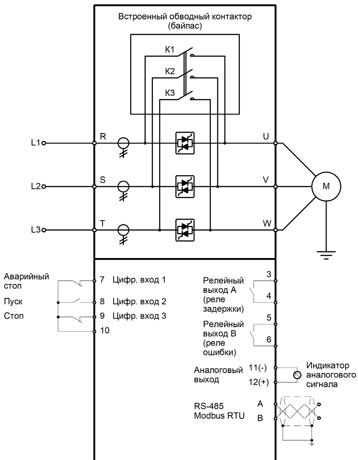
Схема подключения с встроенным обводным контактором для серии SBI
