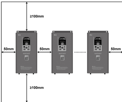
Рис. 7 - Рекомендуемые расстояния при монтаже тормозного модуля
