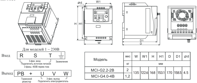
Модель 2 серии MCI
