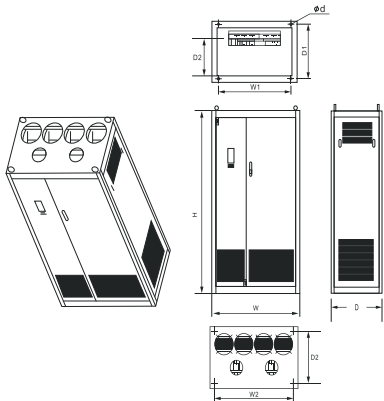
Модель 8 серии FCI
