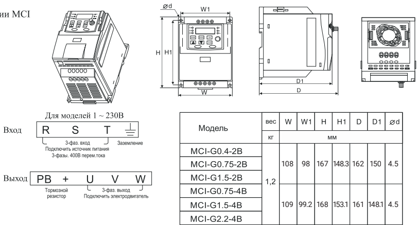
Модель 2 серии MCI
