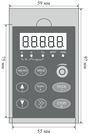
Установочные размеры панели
