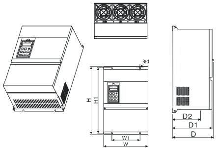
Модель 5 серии FCI
