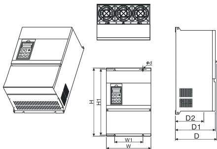
Модель 3 серии FCI
