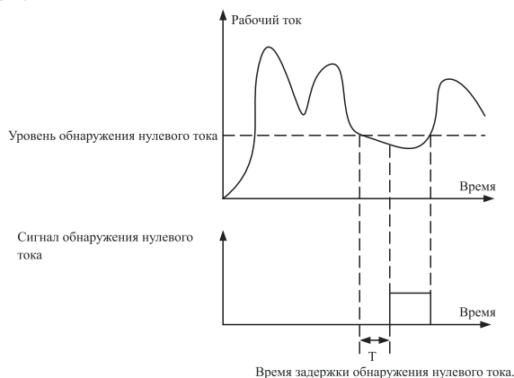
Время задержки обнаружения нулевого тока.
