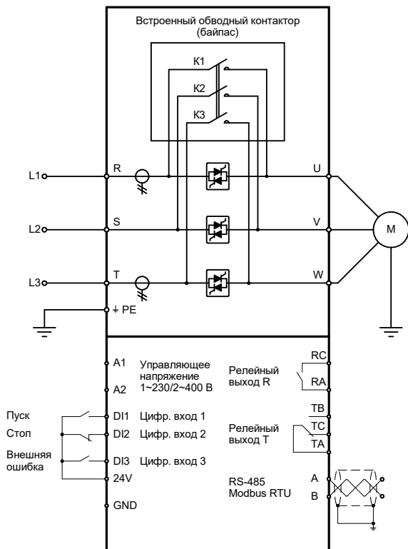
Рисунок 26 – Схема подключения клемм устройства плавного пуска серии SBIM мощностью от 18.5 кВт
