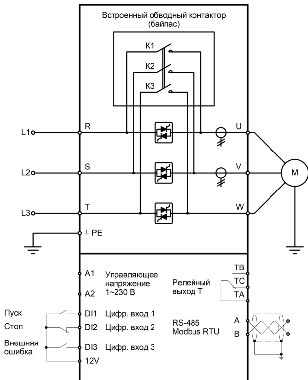
Рисунок 2а – Схема подключения клемм устройства плавного пуска серии SBIM мощностью до 15 кВт
