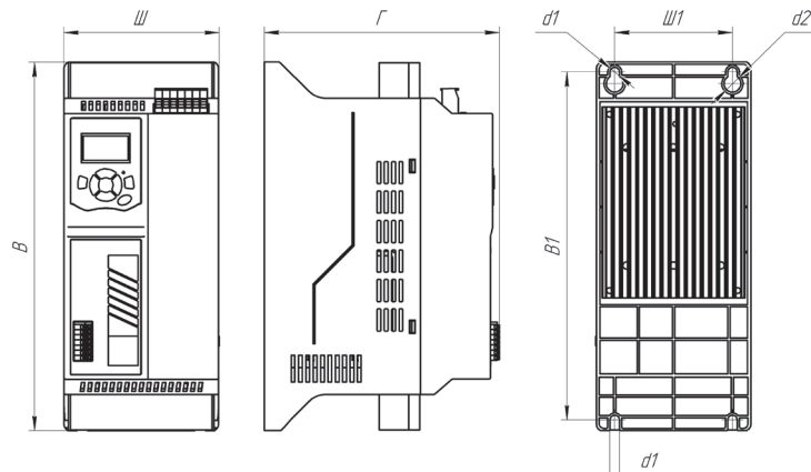
Схема модели серии SBIM (модель мощностью 18,5-37 кВт)
