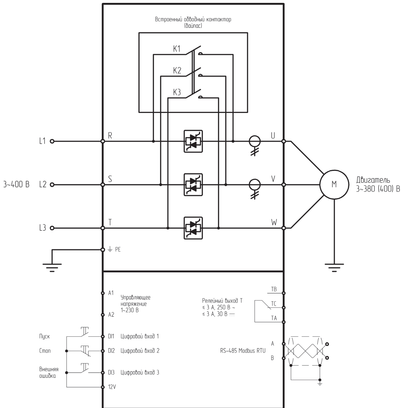
Стандартная конфигурация УПП SBIM мощностью до 15 кВт
