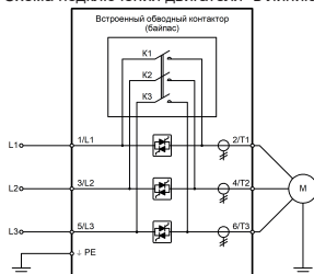
Рисунок 2 – Подключение силовых клемм
