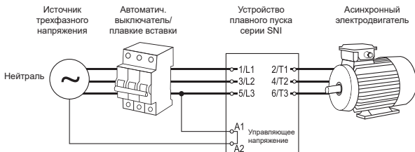
Рисунок 1 – Дополнительное оборудование
