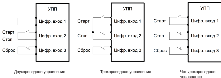
Рисунок 3 – Схемы управления
