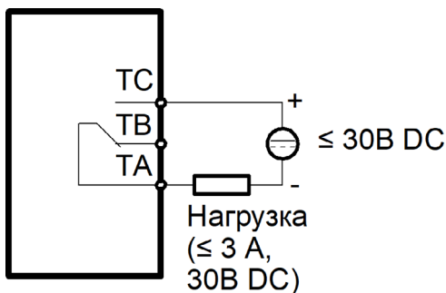
Рисунок 3.13 – Схема подключения нагрузки переменного тока к релейному выходу
