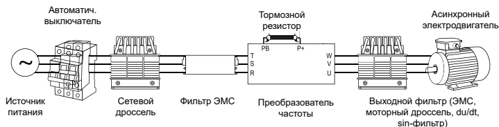
Рис. 1 – Дополнительное оборудование
