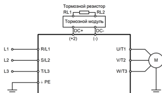
Рис. 3.2.5 Подключение силовых клемм
